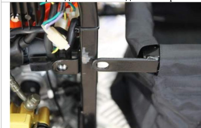
3.11.4. Стыкуем каркас сиденья с рамой моторного блока так, как указано на рисунках.
