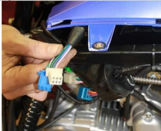
3.1.6. Выводим жгут проводов от приборной панели на левую сторону по ходу движения снегохода.
