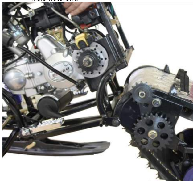
3.9.5. Стыкуем блоки вместе.
