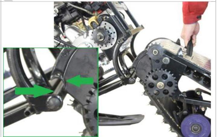
3.9.4. Закинув одной рукой блок двигателя вперед, второй рукой приподнимается гусеничный блок. Заводим полукруглый стыковочный выступ на гусеничном блоке на стыковочную трубу моторного блока.
