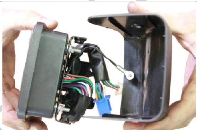
3.1.4. Снимаем декоративную крышку панели приборов.
