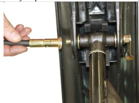
3.6.3. Фиксируем его с помощью болта и гайки из комплекта крепления лыж.
