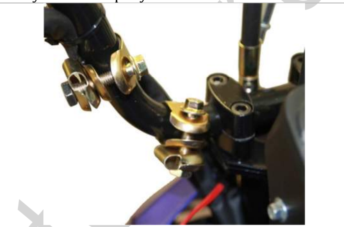
3.15.11. Всего хомуты большой и малый должны быть установлены так как указано на рисунке (с левой и правой сторон снегохода).
