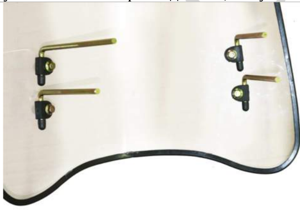
3.15.6. Общий вид установленных кронштейнов на лобовое стекло.
