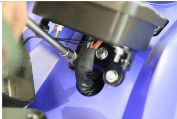
3.1.7. С помощью болтов из комплекта поставки прикручиваем панель приборов
