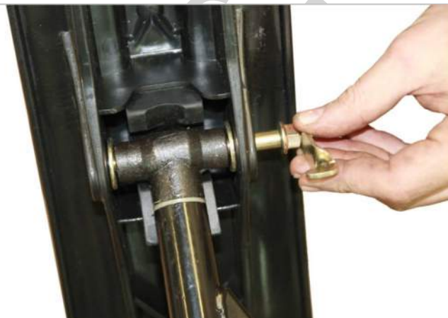
3.6.2. Фиксируем его с помощью болта и гайки из комплекта крепления лыж.
